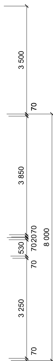
Elevation 1
